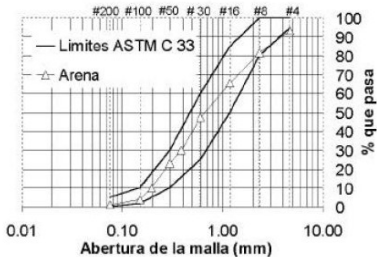
Figura 3. Granulometría de la arena
