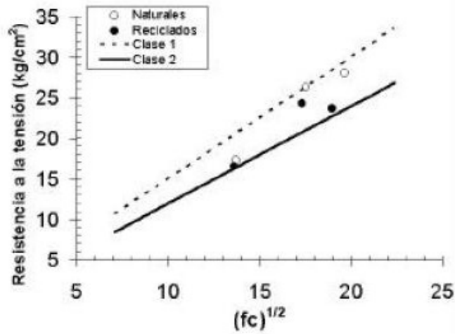
Figura 8. Resistencias a la tensión alcanzadas
