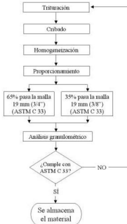
Figura 1. Proceso de fabricación de agregados
