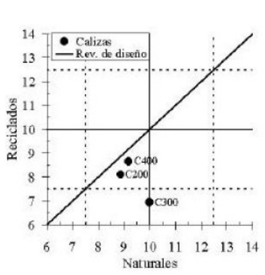
Figura 5. Posicionamiento de revenimientos reciclados-naturales
