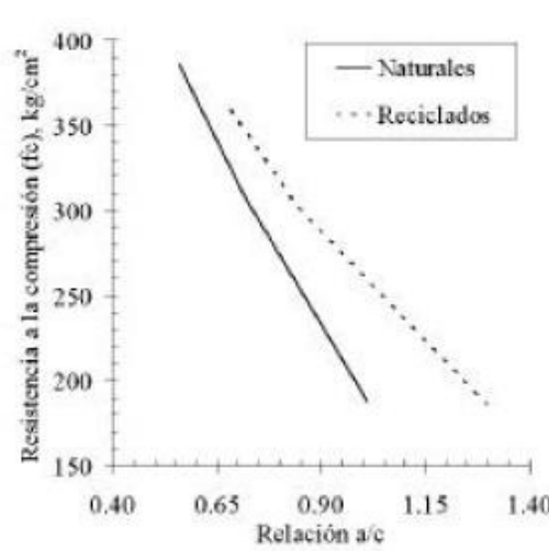
Figura 6. Curvas f_c -relación a/c
