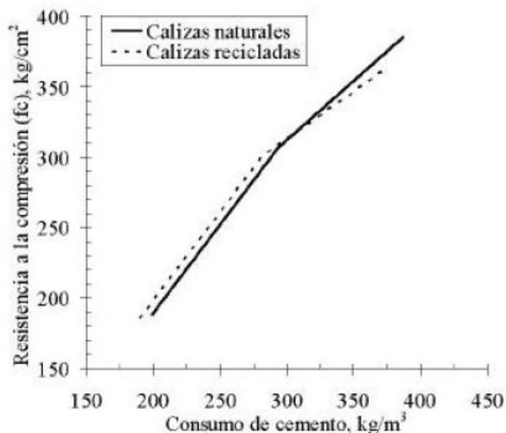
Figura 7. Eficiencia en el consumo de cemento
