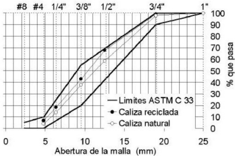
Figura 2. Granulometría de agregados gruesos
